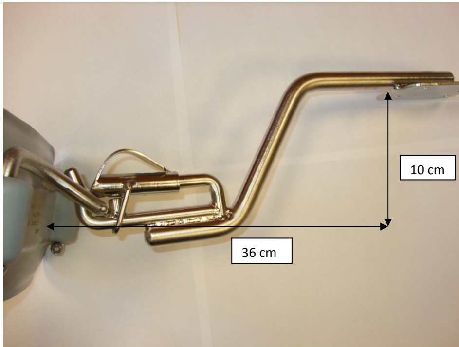
Målskisse av RBD1000S:
